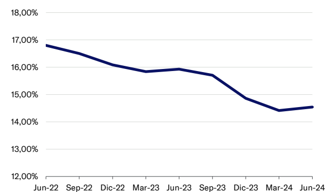
GRÁFICO 6 Comportamiento del IAC
